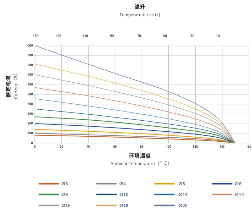
降额曲线—片簧端子
