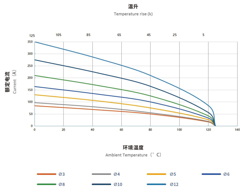
降额曲线—开槽端子
